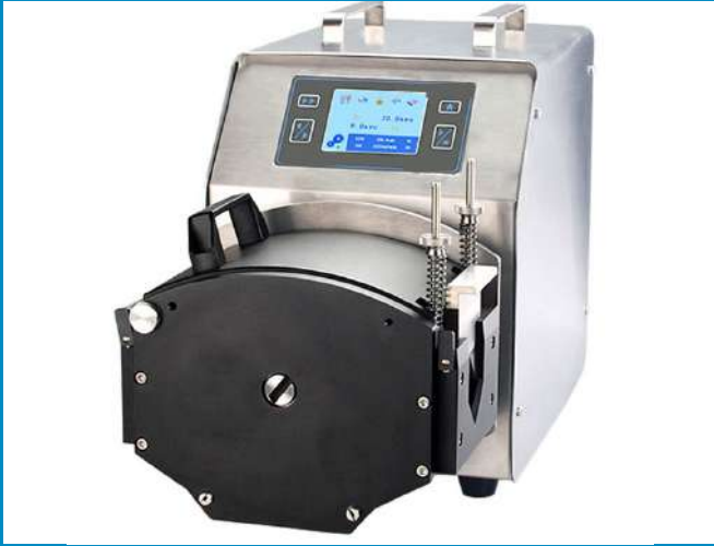
BOMBA DOSIFICADORA LÍQUIDOS Y VISCOSOS BP600
