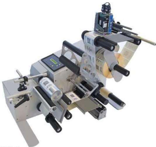
ETIQUETADORA SEMI-AUTOMÁTICA I-LABEL ROUND CILÍNDRICOS
